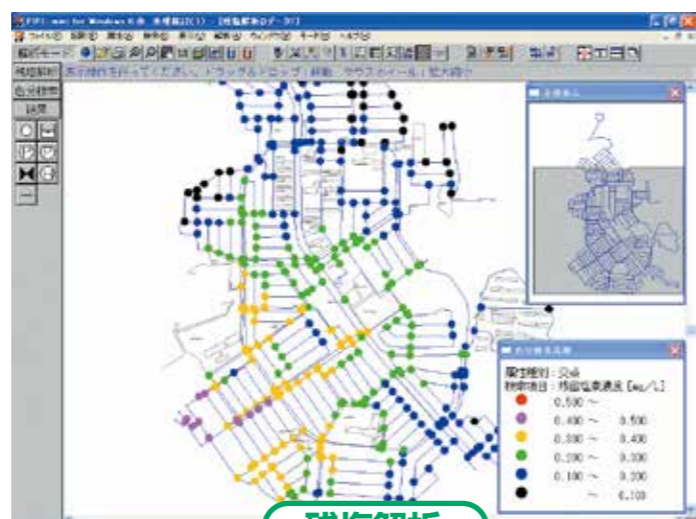
残塩解析
