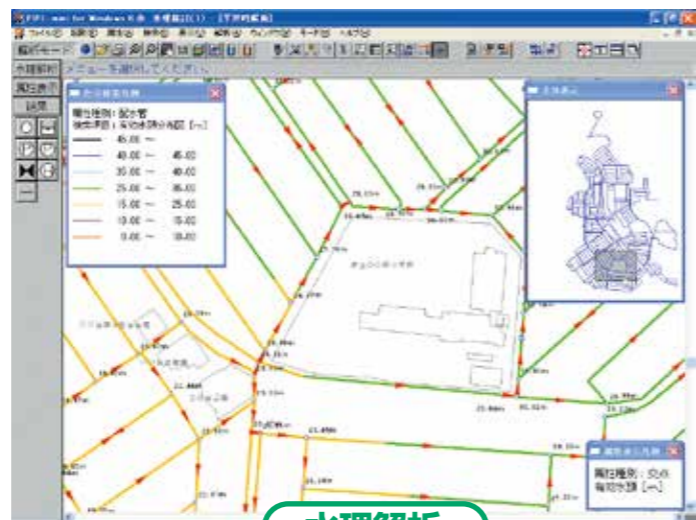
水理解析
