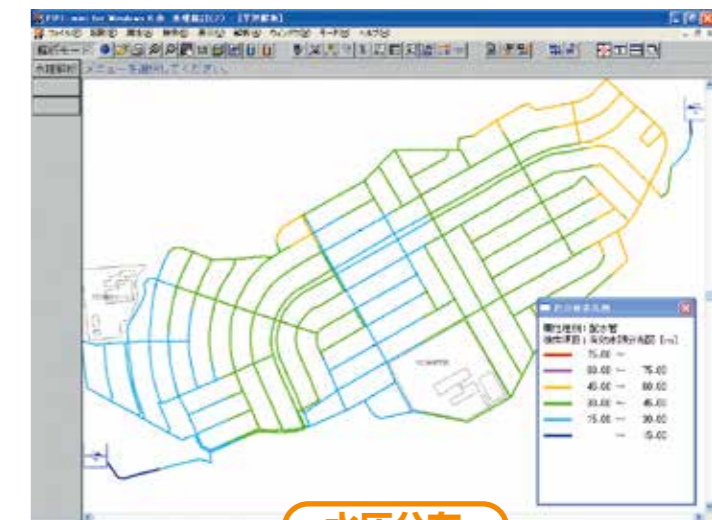
水圧分布
